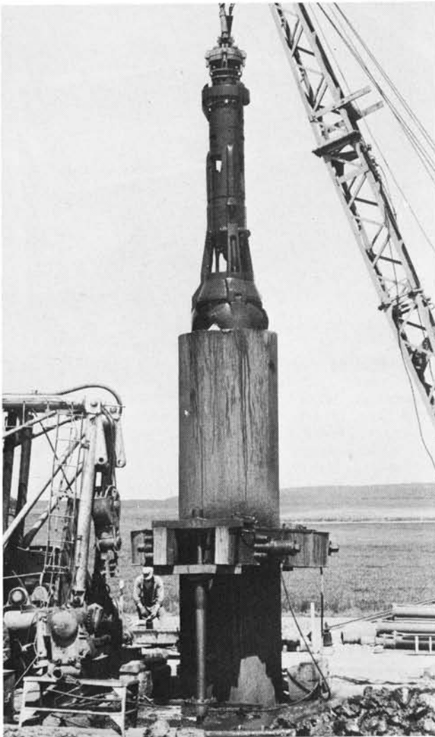
5 Einpressen der Verrohrung ( \varnothing 1220 mm) und Herausfordern des Bohrgutes mit dem Baade-Greifer ( \varnothing 1 m)
