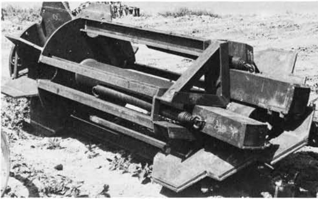
7 Klappmeißel (Durchgang \varnothing 1,1 m, aufgeklappt \varnothing 1,6 m) für das Hinterschneiden unterhalb der Verrohrung
